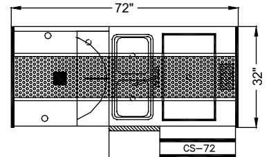
CS-72-CCW (plan view)
